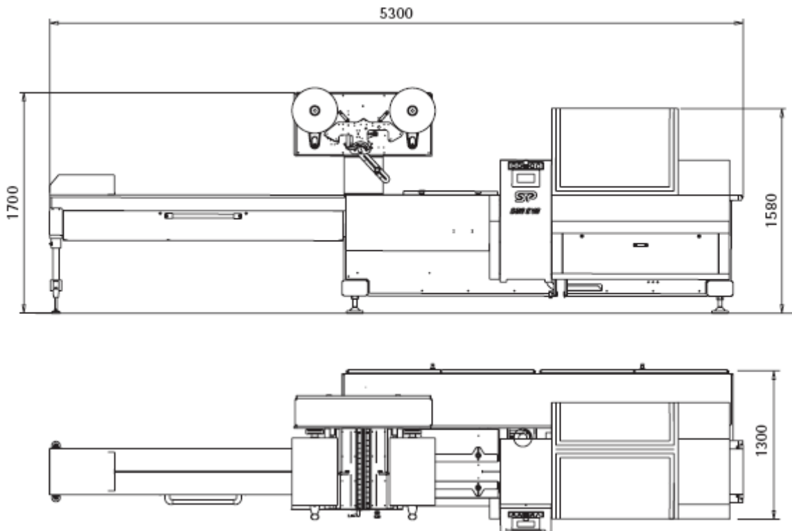
Schema utilaj GSP 600 EVO
