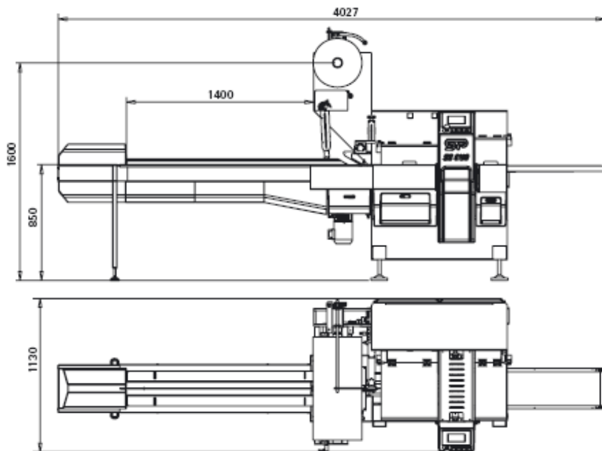
Schema utilaj GSP55 EVO
