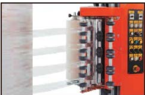
Transport film cu sistem de tăiere longitudinală CP 86 (opțional)
